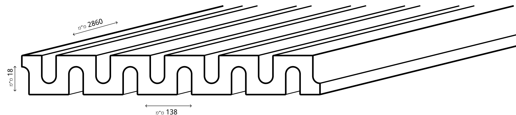
קורות גל
