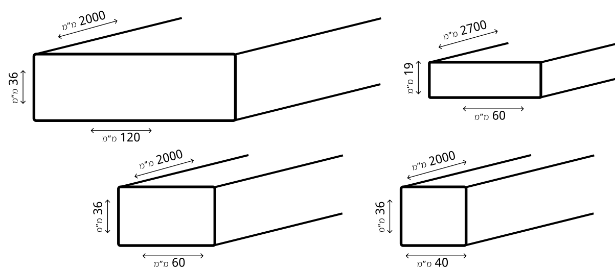
סרגלים
